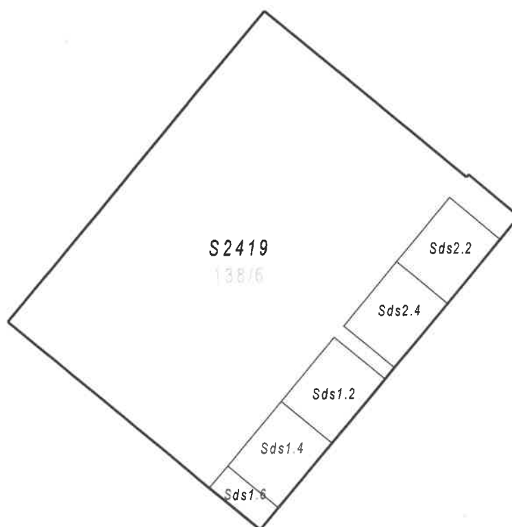
Prikaz sestavine dela stavbe (M = 1:150)
